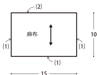
内ポケット 1枚
