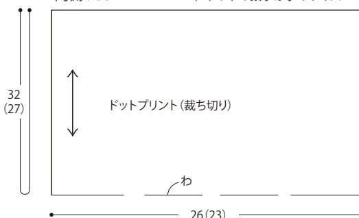
配置図 3ポケットポーチ小 外側(前・後ろ)
