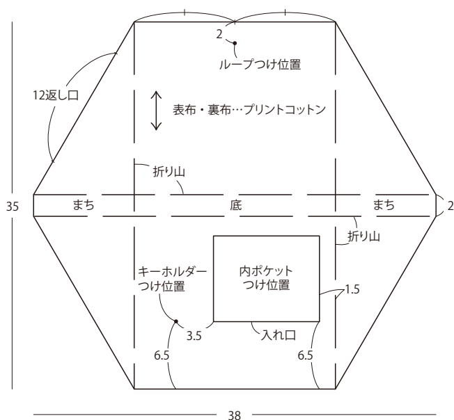
配置図 内側(表布・裏布各1枚)
